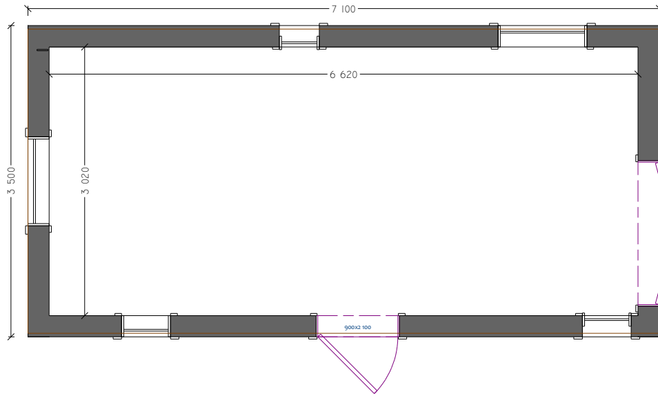
BASMODELL Brutoarea 25 m 2 Bred 3,5m Längd 7,1m Höjd 3,2m
