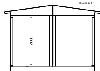
SEKTION
