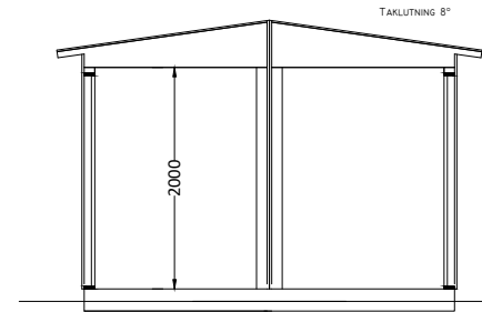
SEKTION
