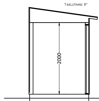
SEKTION
