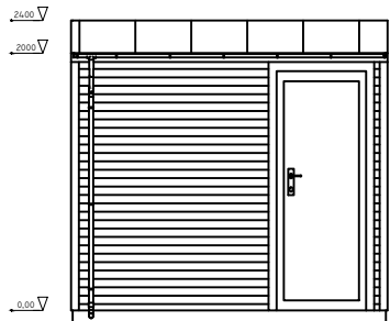
ENTREFASAD
